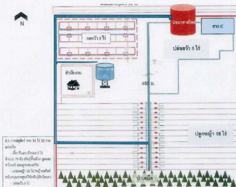
ภาพที่ 3 การวางแผนเดินท่อในพื้นที่แปลงในแปลงปศุสัตว์ พื้นที่ 31 ไร่
